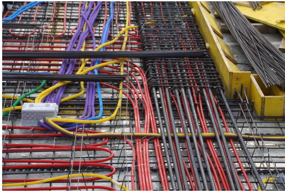
TABS-Verlegung
